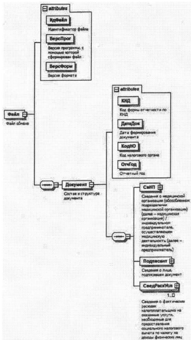
Рисунок 1. Диаграмма структуры файла обмена
